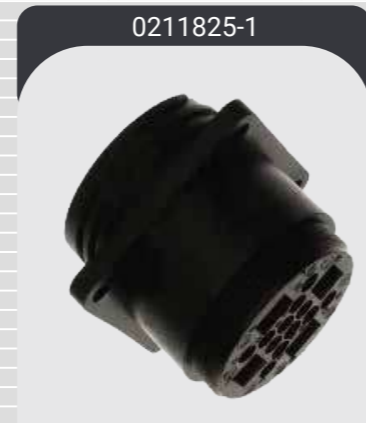
Вилка CPC 23мм, 16 Контактв
